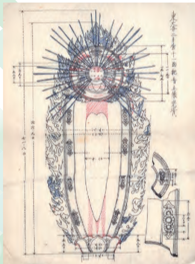
《修理図解 東大寺二月堂》 昭和10～24年頃(c.1935-49) 当館蔵
